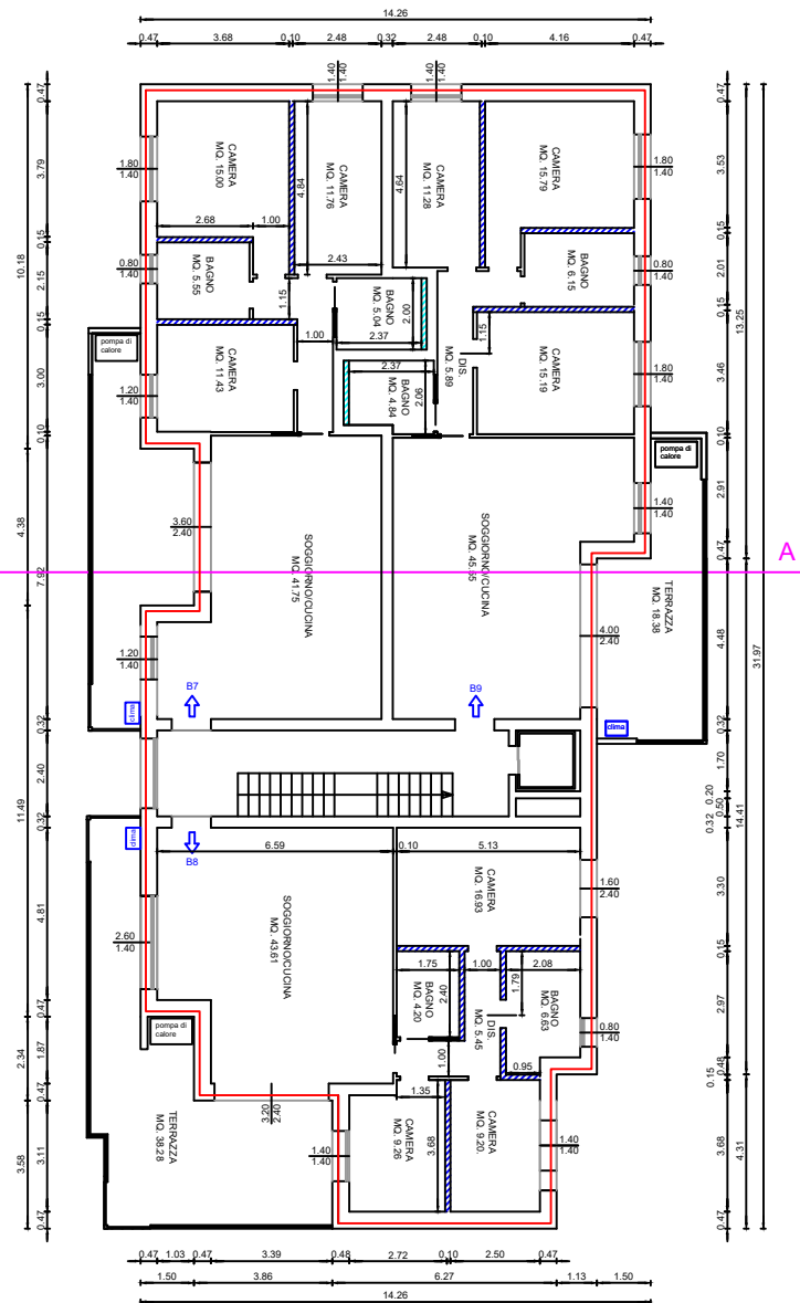
PIANTA PIANO SECONDO
